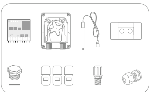
Peristaltische pomp pH-chip Kabelwartel Dop 1/2" Afdichting 1/2" Aansluitstuk sondehouder Sondehouder pH-sonde Set bufferoplossingen
