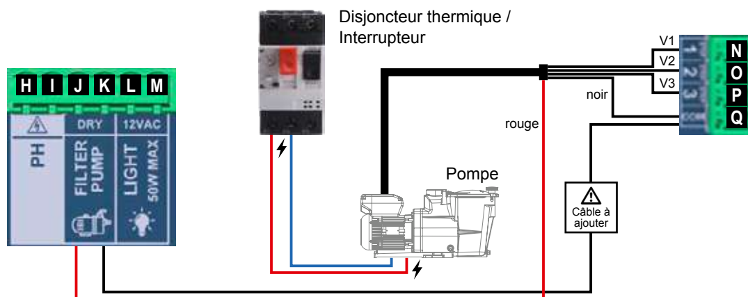
Schéma d'installation d'une pompe à vitesse variable sur l'AquaRite® +
