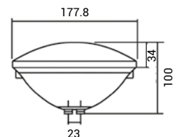
Lampadine (dimensioni in mm)
